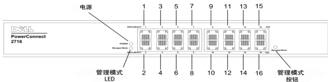
图 2-3. PowerConnect 2716 前面板
