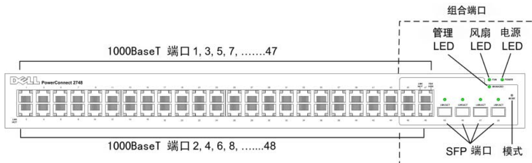
图 2-7. PowerConnect 2748 前面板
